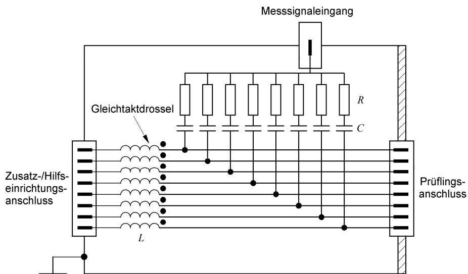
Bild D.5 – Beispiel eines vereinfachten Schaltbildes für ein CDN-T4 für ungeschirmte, symmetrisch betriebene Leitungen (siehe 6.2.1.2)
