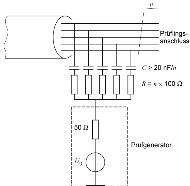
Bild 5c – Prinzip der Einkopplung auf ungeschirmte Leitungen
