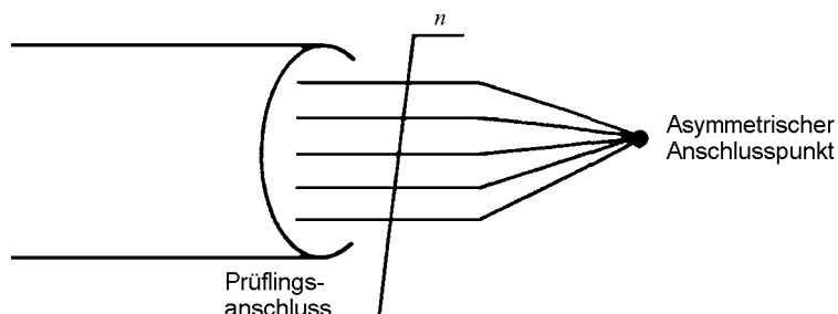
Bild 8a – Festlegung des asymmetrischen Anschlusspunktes bei ungeschirmten Leitungen
