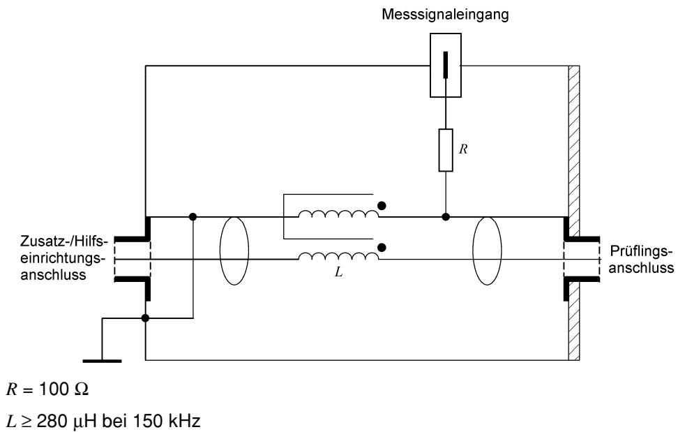
Bild D.1 – Beispiel eines vereinfachten Schaltbildes für ein CDN-S1 für geschirmte Leitungen (siehe 6.2.1)
