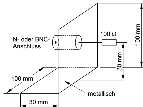
Bild 7c – Prinzip des Aufbaus zur Überprüfung der Einfügungsdämpfung von zwei 150-Ω-zu-50-Ω-Übergängen
