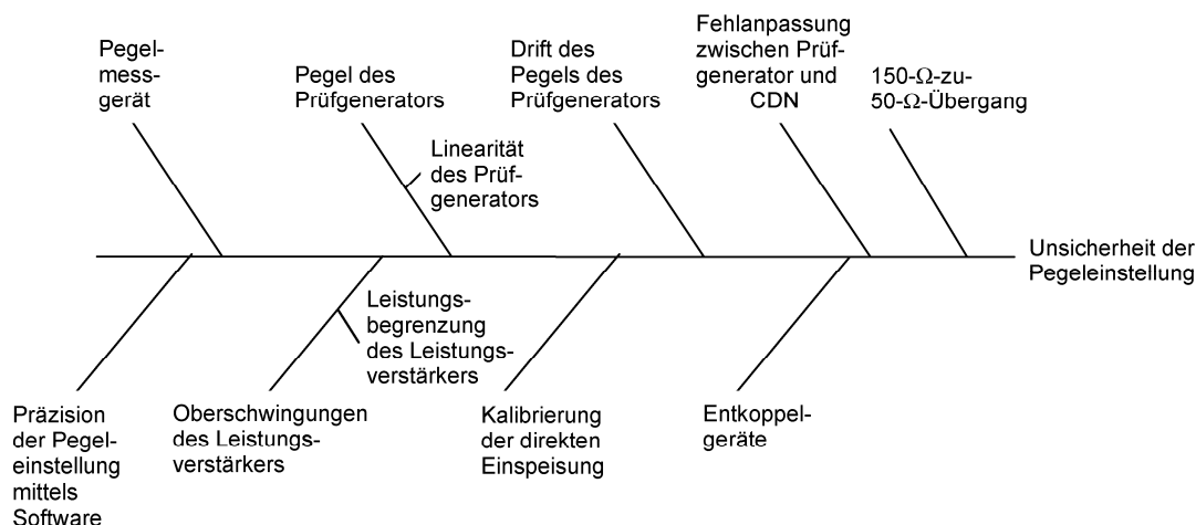
Bild G.4 – Beispiel für Einflüsse auf das Messverfahren bei Verwendung der direkten Einspeisung
