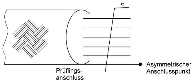
Bild 8b – Festlegung des asymmetrischen Anschlusspunktes bei geschirmten Leitungen
