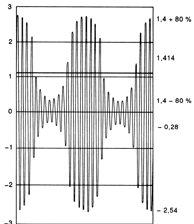
Bild 4b – Moduliertes HF-Signal 80 % AM U_{pp} = 5,09 \text{ V} , U_{rms} = 1,12 \text{ V}
