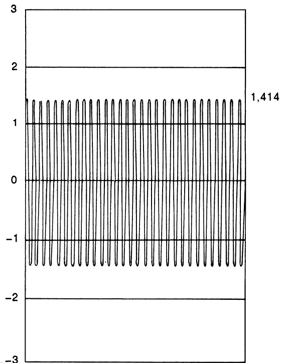
Bild 4a – Unmoduliertes HF-Signal U_{pp} = 2,82 \text{ V} , U_{rms} = 1,00 \text{ V}
