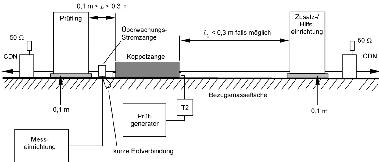
Bild A.6 – Allgemeines Prinzip eines Prüfaufbaus mit Koppelzangen
