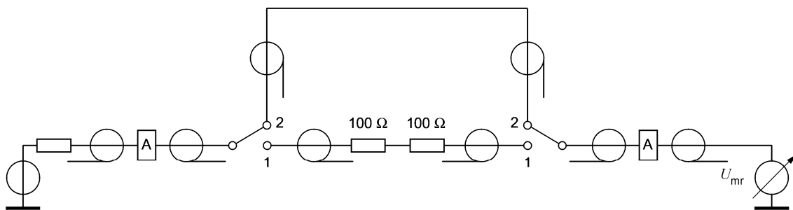
Bild 7b – Prinzip des Aufbaus zur Überprüfung von Z_{ce} der Koppel-/Entkoppelnetzwerke
