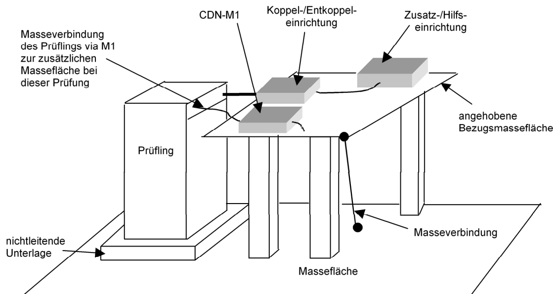
Bild F.1 – Beispiel für den Prüfaufbau mit angehobener horizontaler Bezugsmassefläche zur Prüfung von großen Prüflingen
