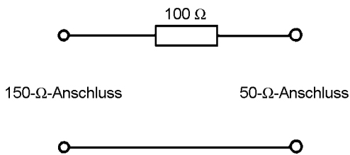
Bild 7c – Prinzip des Aufbaus zur Überprüfung der Einfügungsdämpfung von zwei 150-Ω-zu-50-Ω-Übergängen
