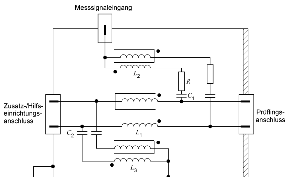
Bild D.3 – Beispiel eines vereinfachten Schaltbildes für ein CDN-AF2 für ungeschirmte, unsymmetrisch betriebene Leitungen (siehe 6.2.1.3)
