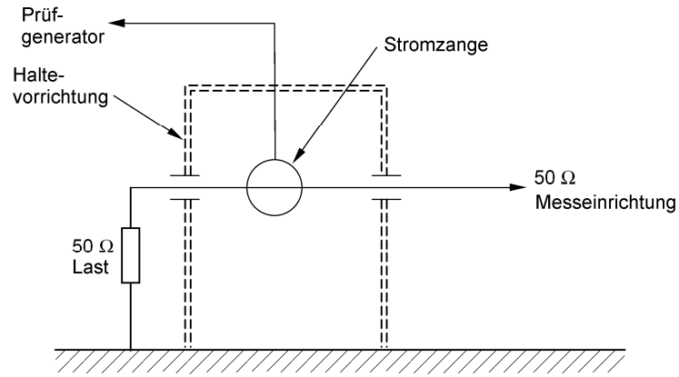
Bild A.1 – Schaltung für die PegelEinstellung in einer 50-Ω-Haltevorrichtung
