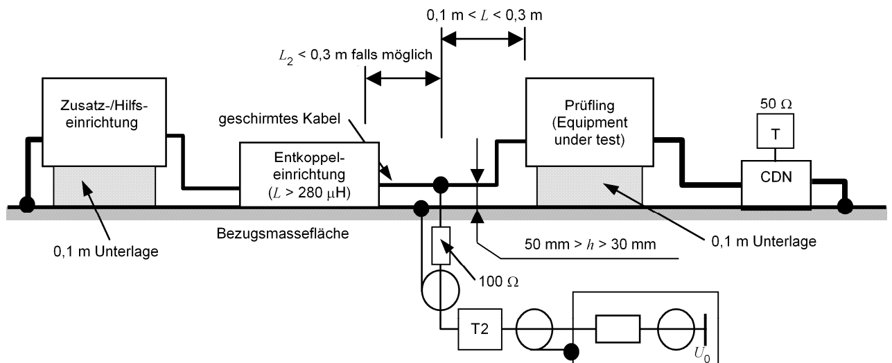
Bild 5b – Prinzip der direkten Einkopplung auf geschirmte Leitungen
