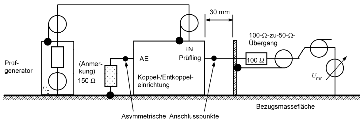
Bild 8b – Festlegung des asymmetrischen Anschlusspunktes bei geschirmten Leitungen
