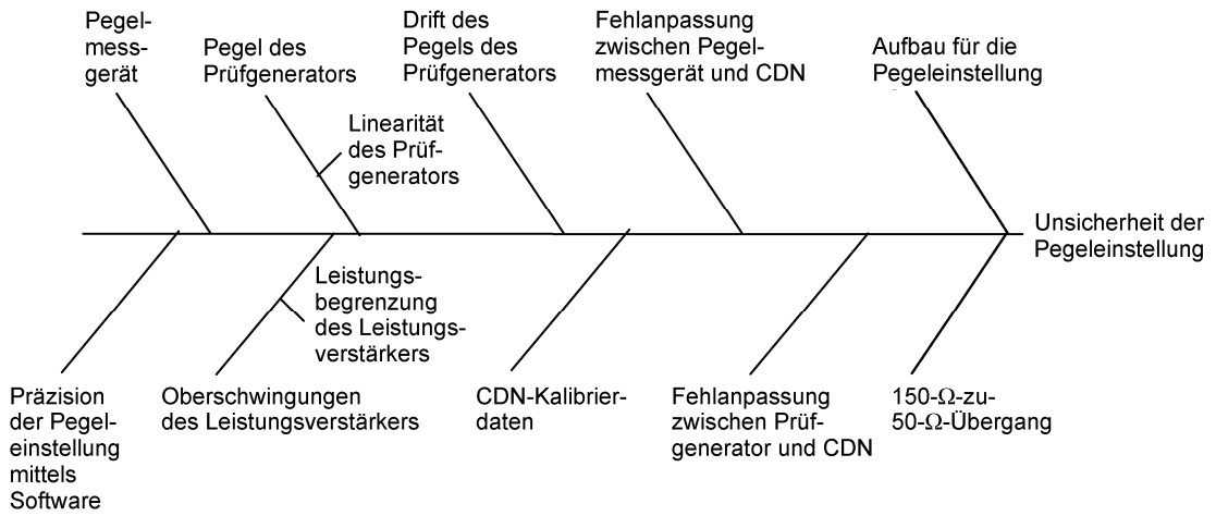
Bild G.1 – Beispiel für Einflüsse auf das Messverfahren bei Verwendung von Koppel-/Entkoppelnetzwerken
