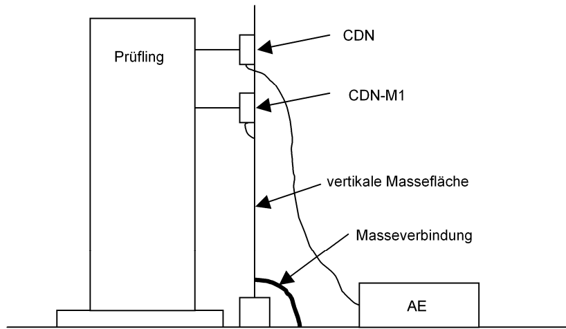
Bild F.2 – Beispiel für den Prüfaufbau mit vertikaler Bezugsmassefläche zur Prüfung von großen Prüflingen
