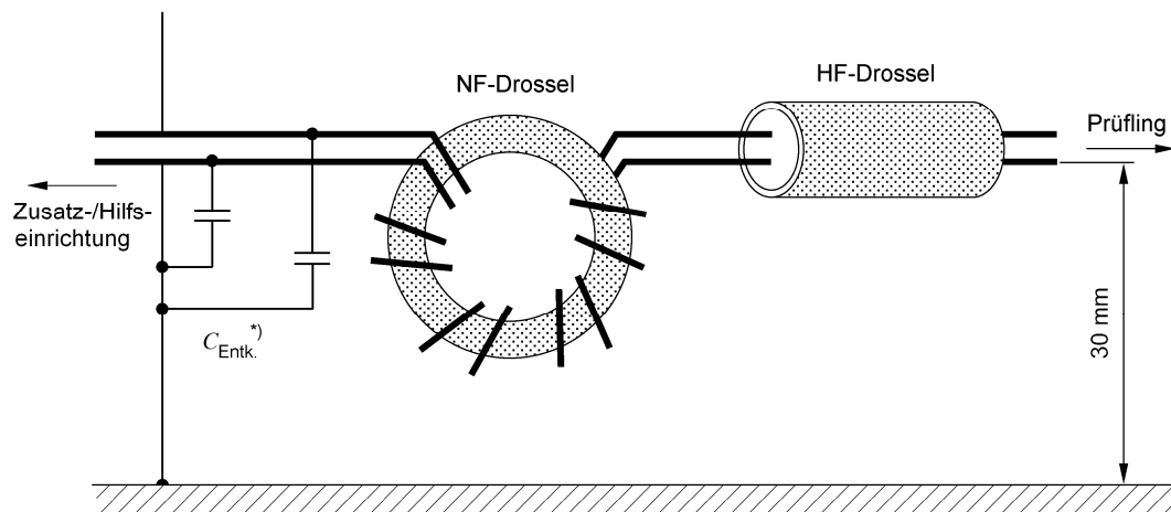
Bild 5c – Prinzip der Einkopplung auf ungeschirmte Leitungen
