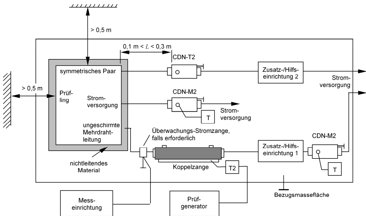
Bild A.6 – Allgemeines Prinzip eines Prüfaufbaus mit Koppelzangen
