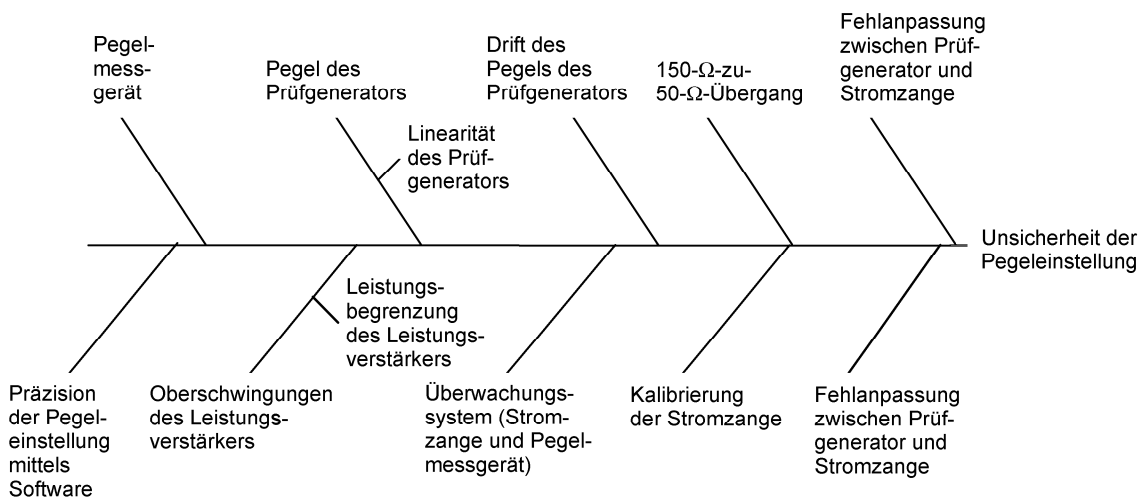
Bild G.3 – Beispiel für Einflüsse auf das Messverfahren bei Verwendung von Stromzangen
