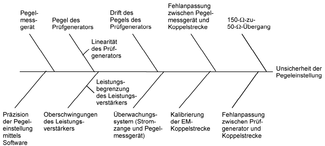
Bild G.2 – Beispiel für Einflüsse auf das Messverfahren bei Verwendung von EM-Koppelstrecken
