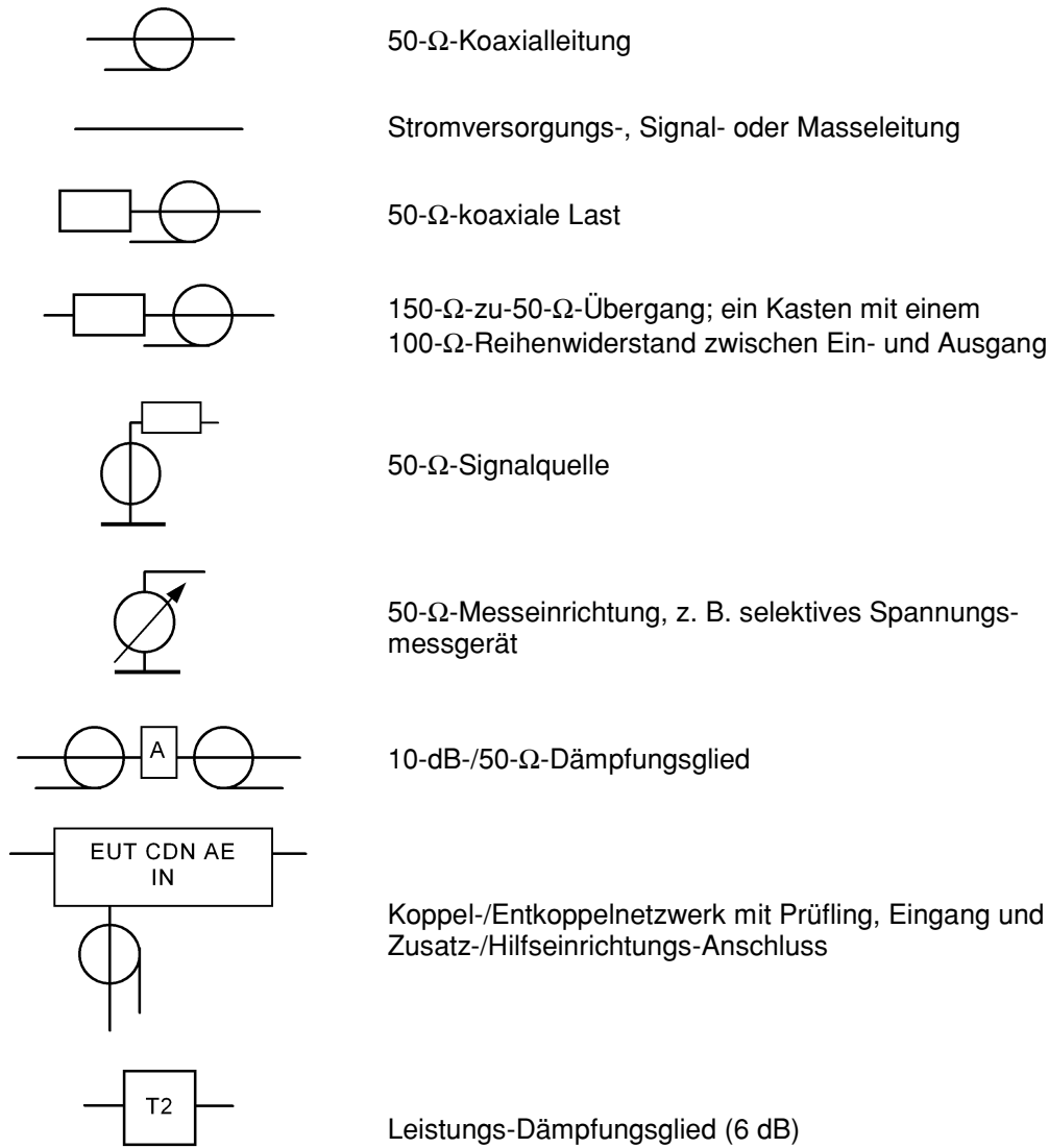
Bild 5a – Liste der in den nachfolgenden Aufbauten verwendeten Symbole
