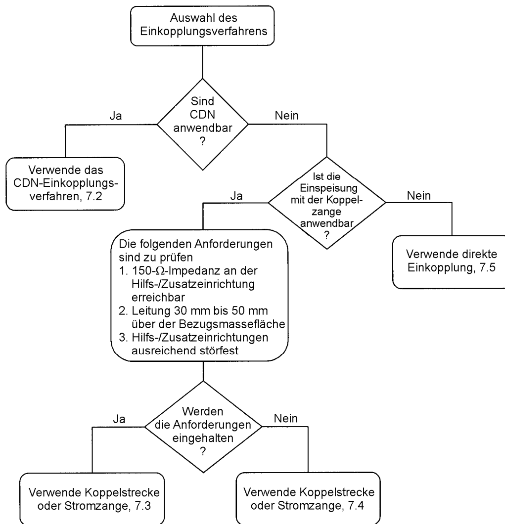
Bild 1 – Regeln für die Auswahl des Einkopplungsverfahrens
